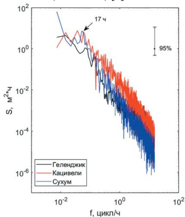
Рис. 7. – Частотные спектры внутренних волн для трёх типов черноморского шельфа – геленджикского (пологий), крымского (приглубый) и абхазского (крутой) (по: [1, рис. 6]). Вертикальными пунктирными линиями отмечены локальные инерционные частоты каждого района.
