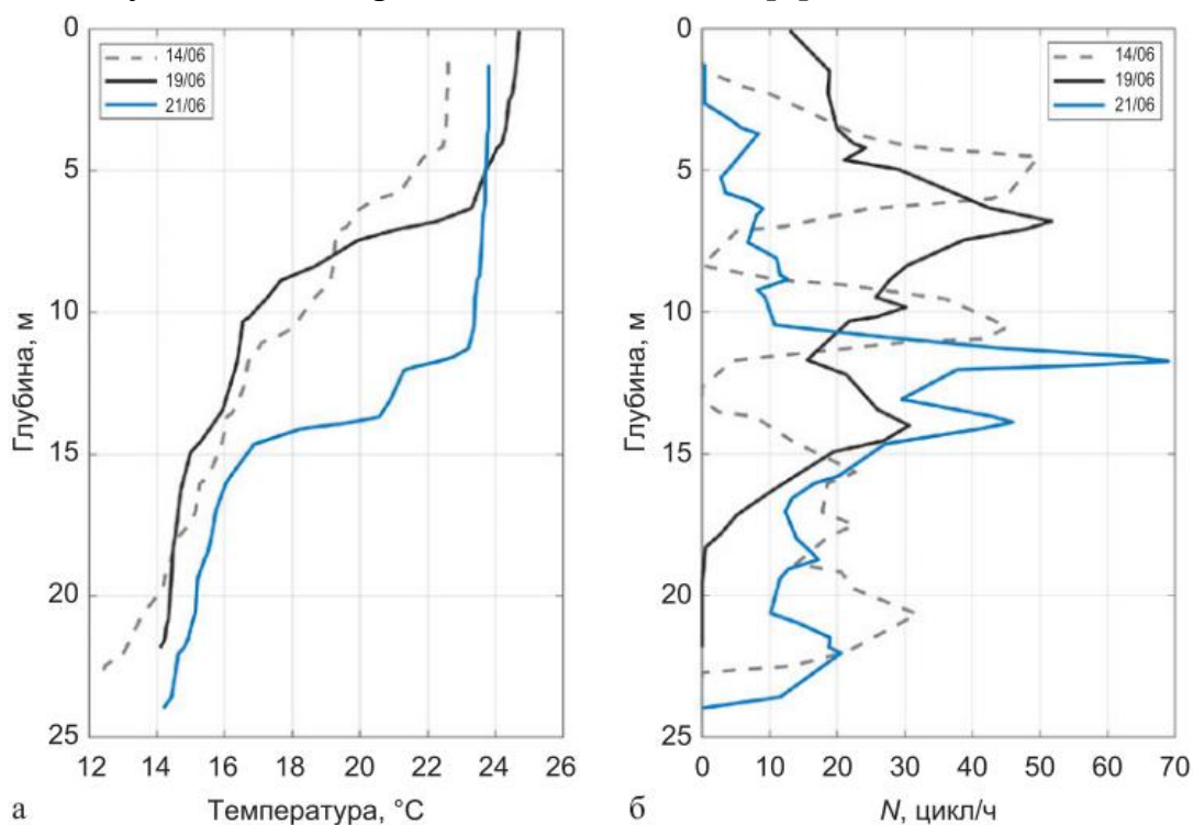
Рис. 6. – Вертикальные профили температуры (а) и частоты Вьяйсяля–Брента (б) по данным STD-зондирований 14, 19 и 21 июня 2023 г. (по: [6, рис. 3]). Хорошо видна эволюция стратификации: углубление ВКС и рост N_{max} к 21 июня.
