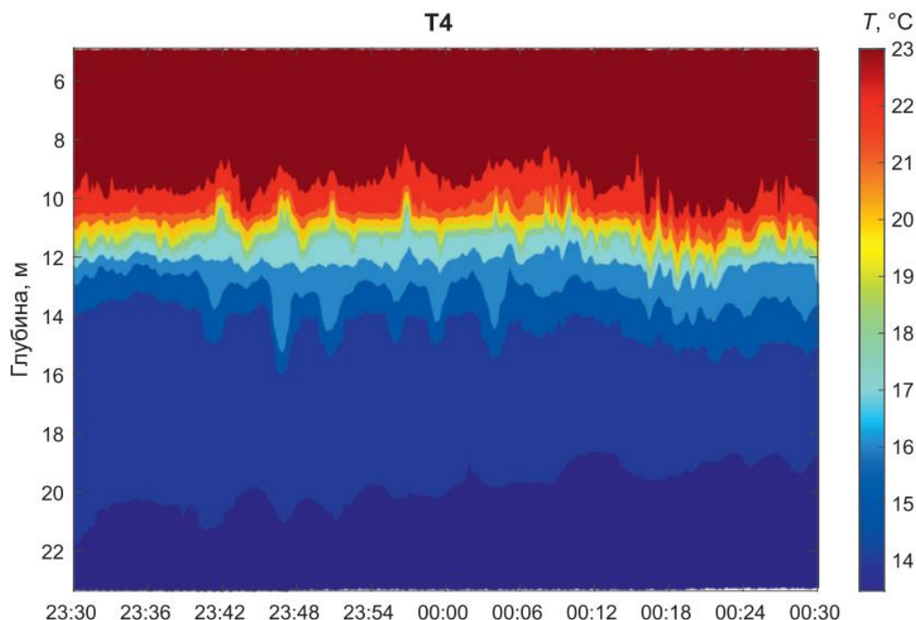
Рис. 10. – Проявление короткопериодных внутренних волн второй вертикальной моды 20–21 июня 2023 г. по данным термокосы T4 (по: [6, рис. 9]).
