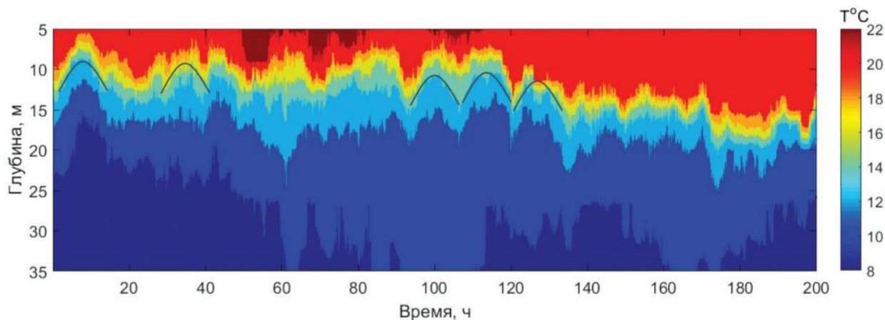
Рис. 8. – Временная изменчивость температурной структуры моря на геленджикском шельфе с 29 мая по 7 июня 2013 г. (по: [1, рис. 2]). Видны 17-часовые колебания термоклина, обусловленные инерционными волнами (выделены тонкими линиями).
