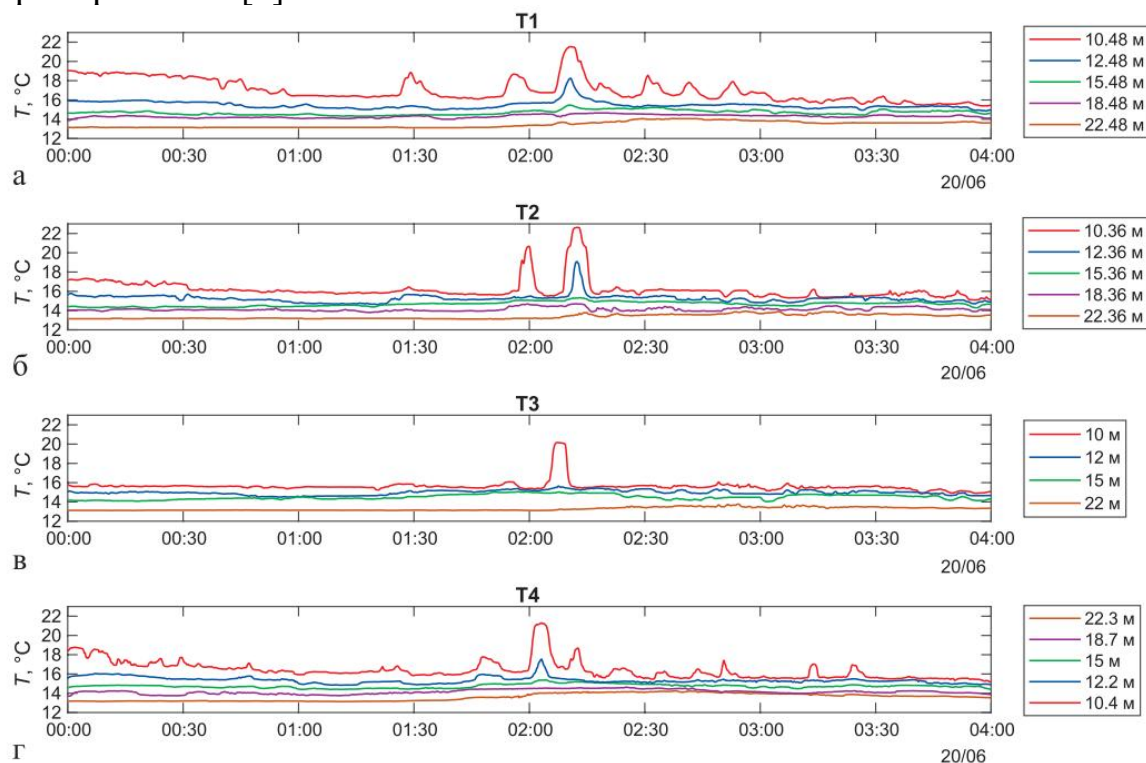
Рис. 9. – Колебания температуры на горизонтах термоксы Т1–Т4 при прохождении цуга внутренних волн первой моды 20 июня 2023 г. (по: [6, рис. 7]). Цветом обозначены горизонты расположения датчиков температуры.
