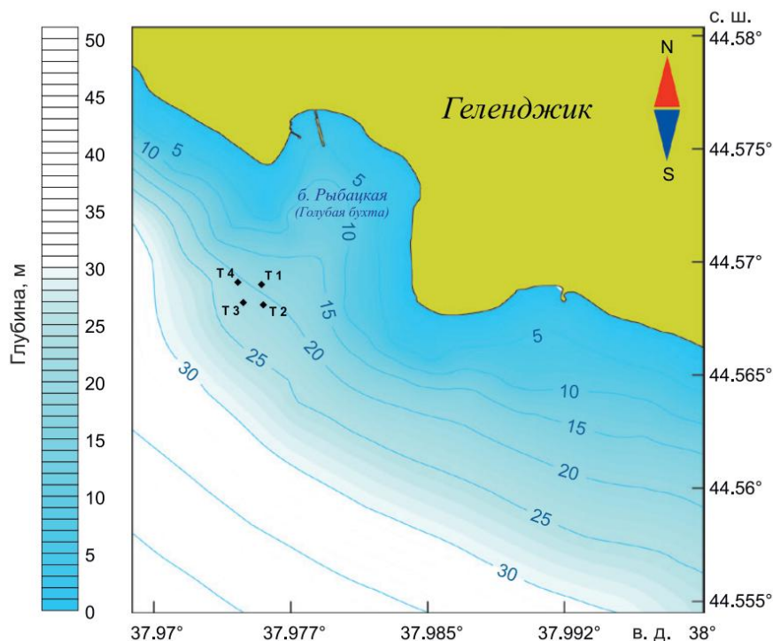
Рис. 1 – Положение заякоренных термокос на карте батиметрии [6].
