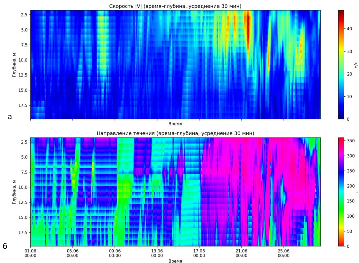
Рис. 17. – Временная изменчивость скорости течения |V| (а) и его направления (б) по данным ADCP (усреднение 30 мин).
