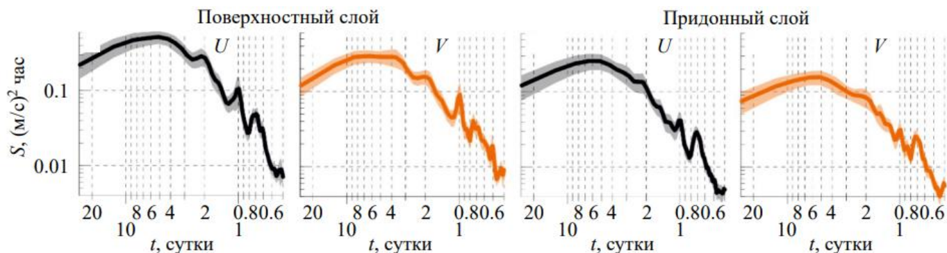
Рис. 5. – Осреднённые частотные спектры компонент U и V скорости течений в поверхностном и придонном слоях по данным ADCP за 2016–2023 гг. (по: [8, рис. 9]). Выделены пики на инерционном ( \sim 17 ч), суточном и синоптических ( \sim 2,2 и \sim 5 суток) периодах.
