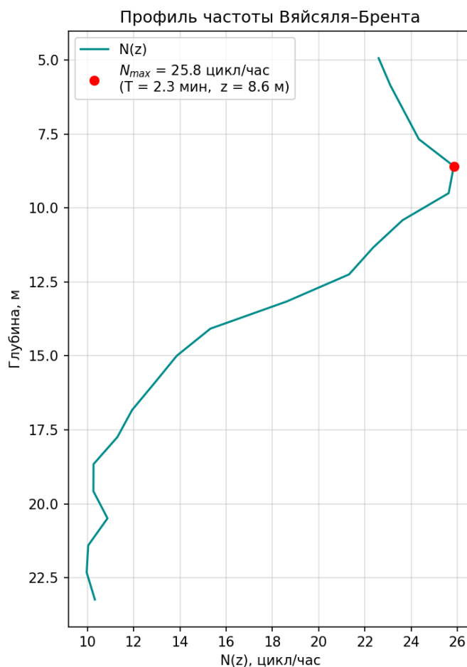
Рис. 3. – Профиль частоты Вяйсяля-Брента с указанным максимальным значением 25.8 цикл/час, период T=2.3 мин.
