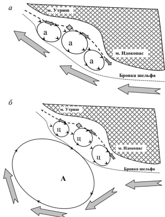
Рис. 4.— Схема формирования субмезомасштабных вихрей на узком северокавказском шельфе (по: [11, рис. 6]): а – при прижатом к склону ОЧТ (СЗ течение) за мысами образуются антициклоны; б – при антициклоническом меандре ОЧТ (ЮВ течение) в зоне сдвига скорости формируются циклоны.
