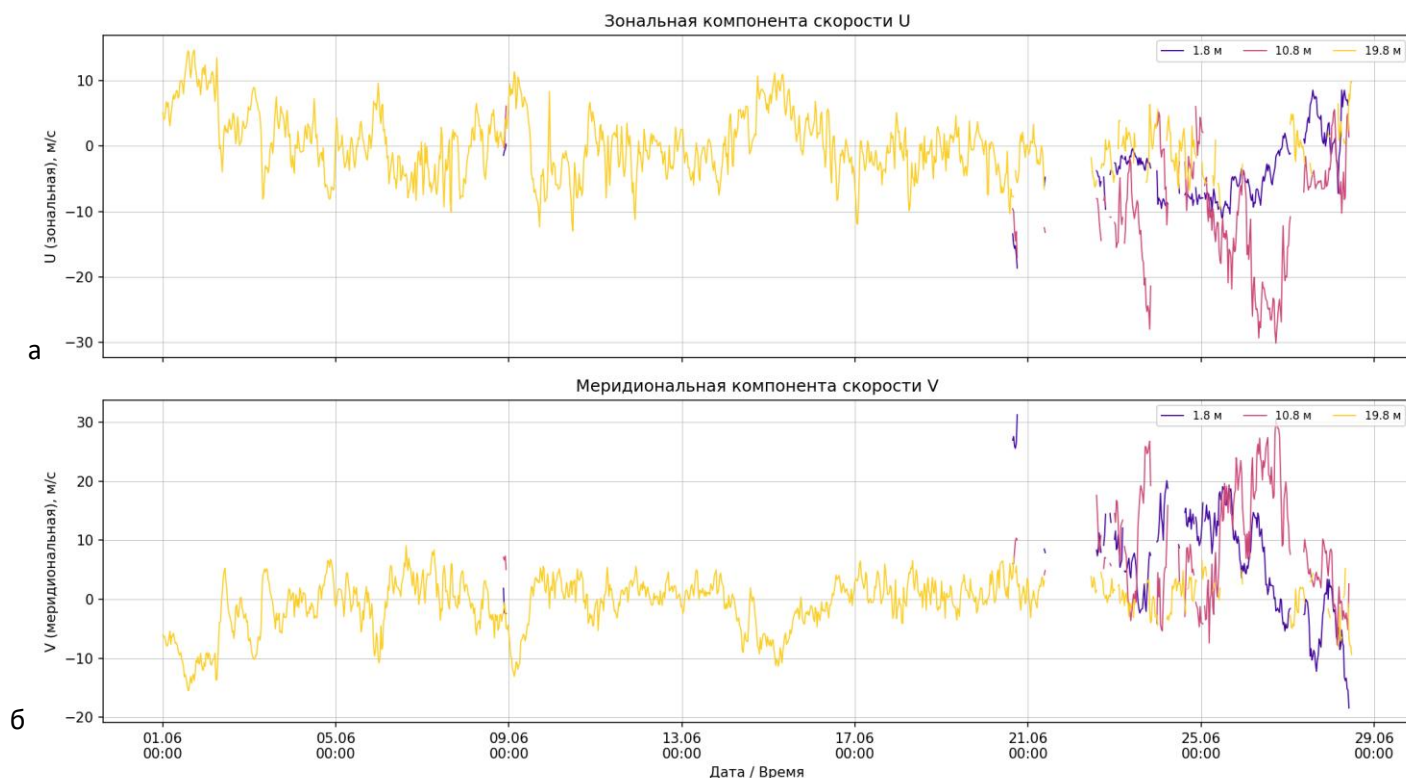
Рис. 19. – Временные ряды зональной U (а) и меридиональной V (б) компонент скорости на горизонтах 1,8; 10,8; 19,8 м (30-мин осреднение).
