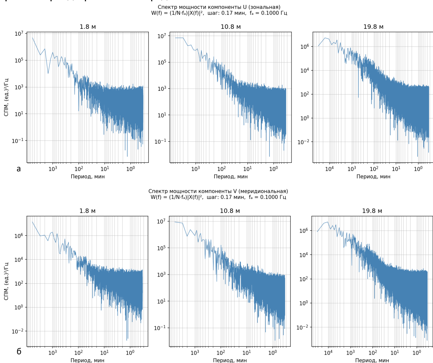
Рис. 23. – Объединённые спектры мощности: (а) – зональная компонента U, (б) – меридиональная компонента V. Горизонты измерений: 1,8 м, 10,8 м, 19,8 м. Представлены периодограммы, по оси абсцисс – период (минуты), по оси ординат – спектральная плотность мощности.
