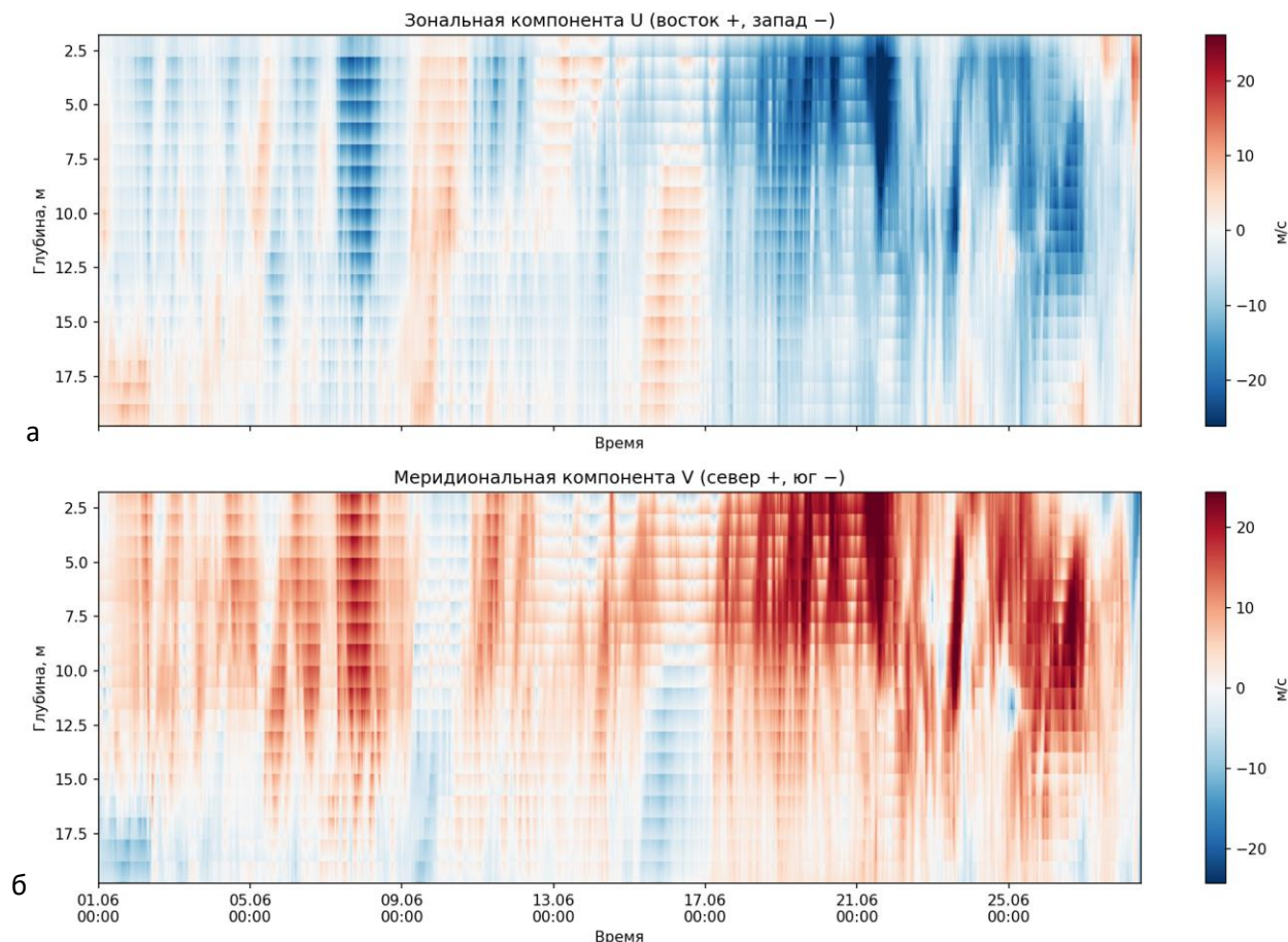
Рис. 18. – Поле временной изменчивости для зональной компоненты U (а) и меридиональной V (б). Усреднение 30 мин, красный – положительные значения (восток/север), синий – отрицательные (запад/юг).
