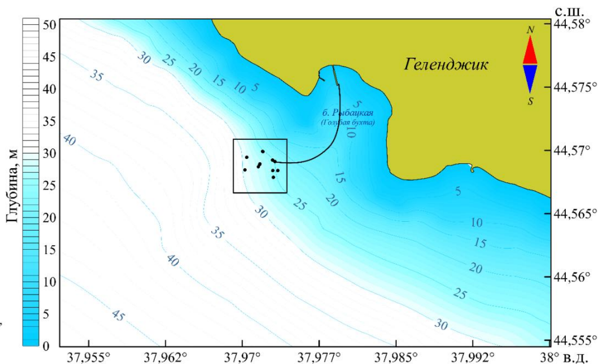
Рис. 29. – Схема расположения термокос в акватории Голубой бухты по данным работы [22] (воспроизведено по: Очередник, Зацепин, 2023). Кружки – точки постановки термокос; глубина в точках постановки 22–23 м. Расположение соответствует полигону настоящего исследования.
