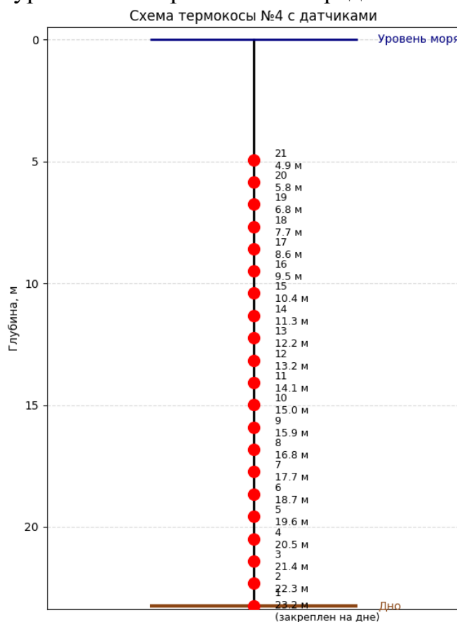
Рис. 11. – Схема термокосы Т4 с отмеченными датчиками (красный) и их медианными глубинами.
