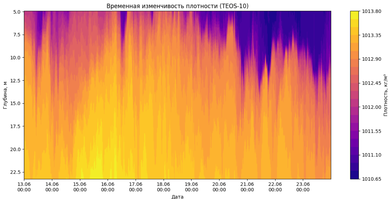
Рис. 2. – Поле временной изменчивости плотности.
